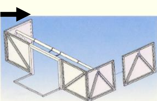
zweite Ecke zusammenschrauben
