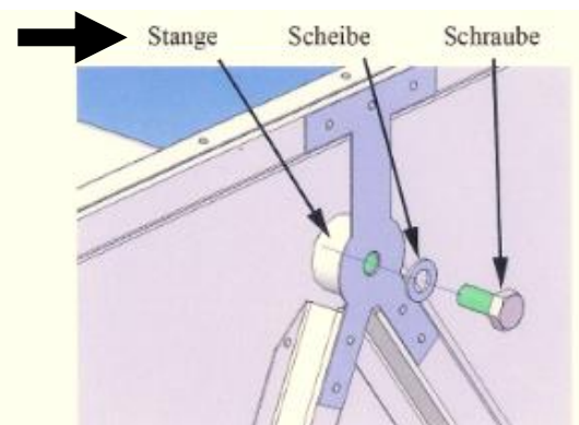
Stange an Beiden Enden an Banden anschrauben
