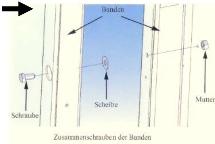
immer je eine Stange mit Gewinde und eine Stange ohne Gewinde zusammenschrauben
