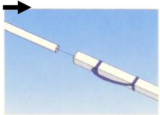
dann je ein rechteckiges Rohr über eine FEST zusammengeschaubte Stange
