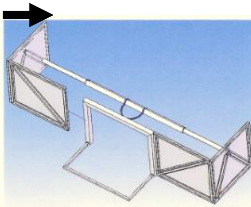
erste Stange an erster Ecke einsetzen, dann zweite Ecke ranschieben und and Tor festschrauben
